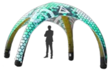
Maße: 4x4 m/ Kombi 8x4 m Höhe 2.45 m Rohrdurchmesser ca. 27 cm Dimensions: 4x4 m/ combi 8x4 m Height 2.45 m Pipe diameter about 27 cm
